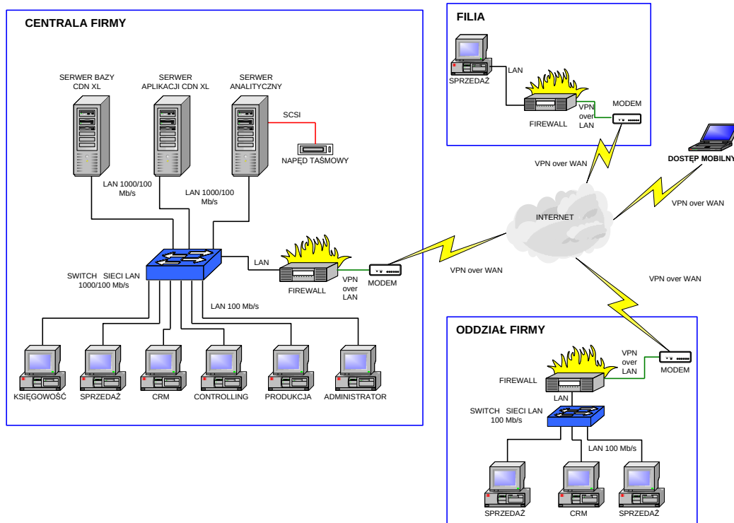
Rysunek 5. Schemat infrastruktury systemu COMARCH ERP XL z uwzględnieniem rozdzielania bazy transakcyjnej, bazy OLAP i usług terminalowych na odrębne serwery.
