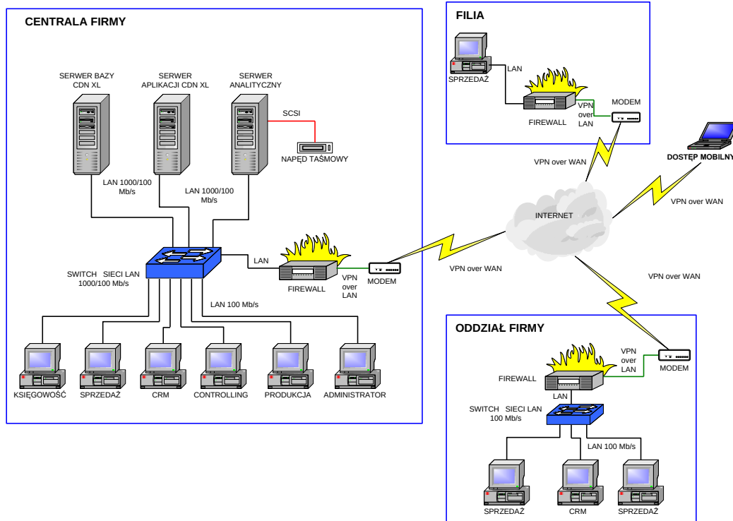
Rysunek 5. Schemat infrastruktury systemu COMARCH ERP XL z uwzględnieniem rozdzielnie bazy transakcyjnej, bazy OLAP i usług terminalowych na odrębne serwery.
